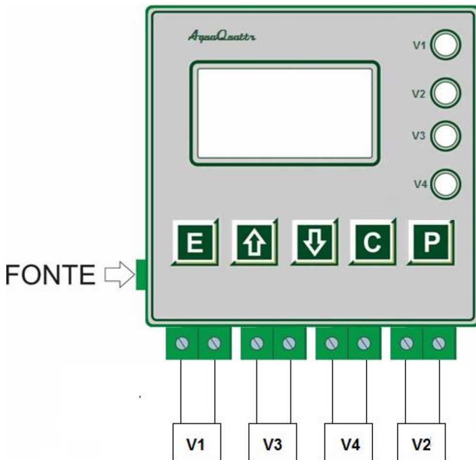
Figura 2 – Configuração de instalação do AquaQuattro.
